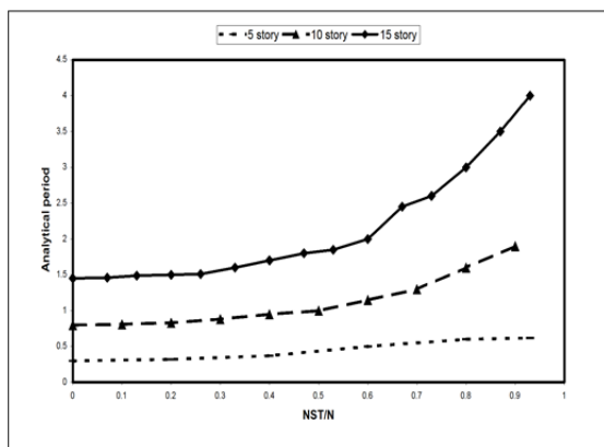
شکل ۵- پریود تحلیلی مود اول سازه‌های ترکیبی
