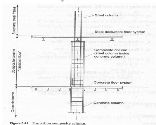
شکل ۲- طبقه انتقالی
