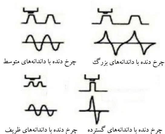
شکل ۹- فرم عمومی قرار گرفتن دندانه‌های روتور و سیگنال خروجی
