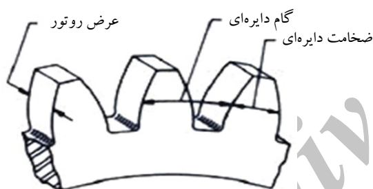
شکل ۸- تصویر برش خورده روتور با ماده مغناطیسی
