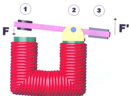
شکل ۱- ساختار کلی و شماتیک یک رله جذبی
