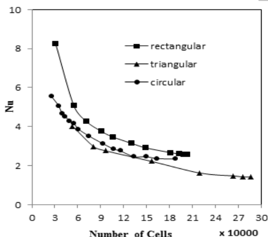
شکل ۳- تغییرات نوسلت متوسط بر حسب تعداد سلول برای هر سه نوع دندان‌ها
