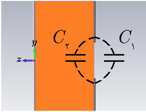
شکل ۱۳- خازن‌های تشکیل شده در مرز پیچ بین دی‌الکتریک و هوا.
