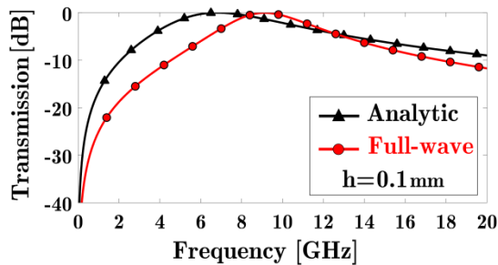
شکل ۱۴- مقایسه نتایج حاصل از شبیه‌سازی تمام موج و تحلیلی ضریب انتقال بدون عبارت G در فرمول‌ها به ازای h = 0.1 \text{ mm}
