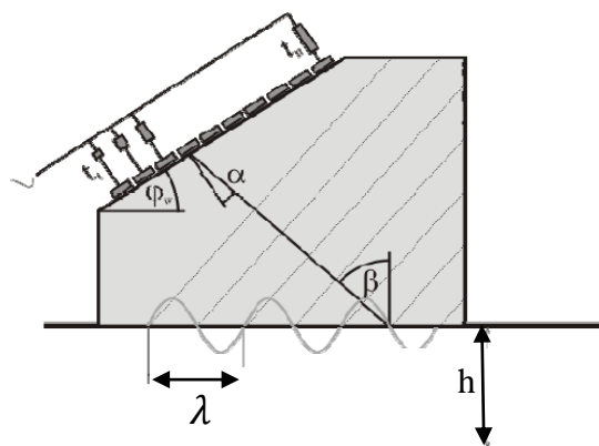
شکل ۳- استفاده از روش آرایه فازی برای تحریک یک مود خاص در ورق
