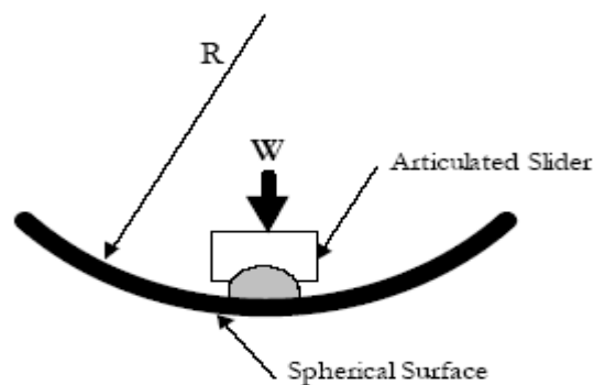
شکل ۵- سیستم آونگ اصطکاکی [۷]
