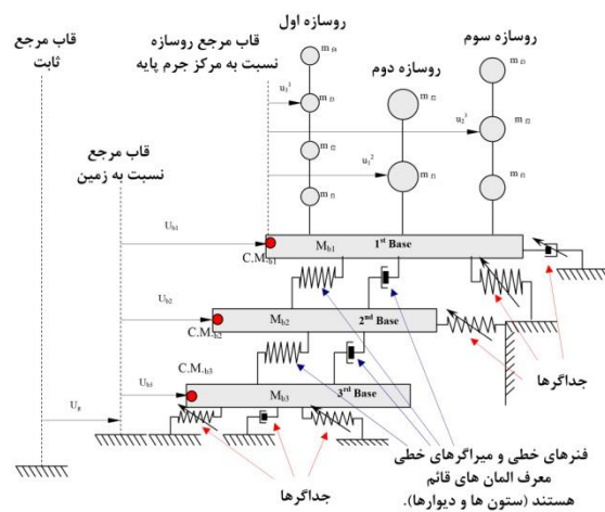
شکل ۳- فرم شماتیک فرضیات مدل سازی سیستم جداساز لرزه ای [۲۰]
