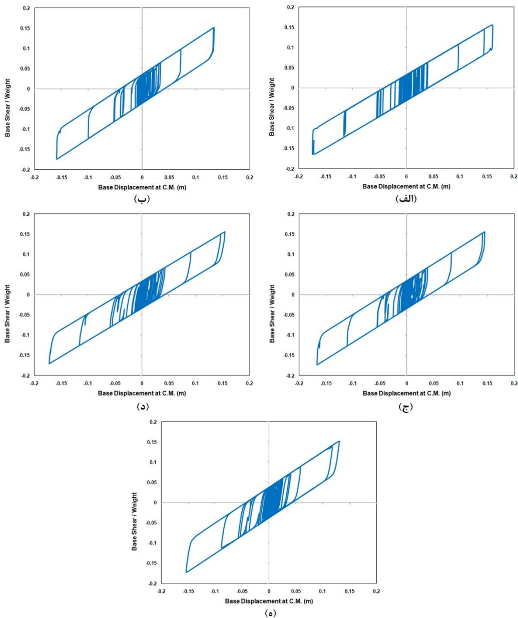
شکل ۶- پاسخ هیستریزیس مدل با نسبت الف- ۱۰۰ درصد جداگر آونگ اصطکاکی ب- ۷۵ درصد جداگر آونگ اصطکاکی ج- ۵۰ درصد جداگر آونگ اصطکاکی د- ۲۵ درصد جداگر آونگ اصطکاکی ه- بدون جداگر آونگ اصطکاکی
