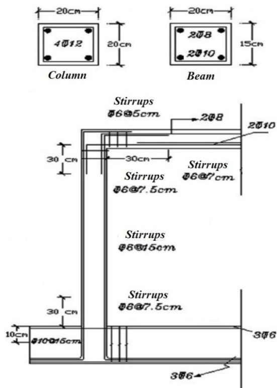
شکل ۶- جزئیات مربوط به قاب آزمایشگاهی همتی [۱۸]
