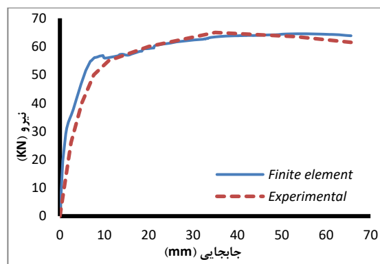
شکل ۷- صحت‌سنجی مدل عددی (اجزای محدود) با مدل آزمایشگاهی
