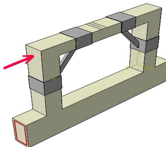
شکل ۷- تصویر قابی که در نرم‌افزار مدل‌سازی شده و محل اثر نیروی جانبی
