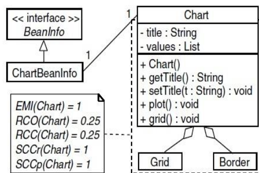
شکل (۳): نمودار کلاس
