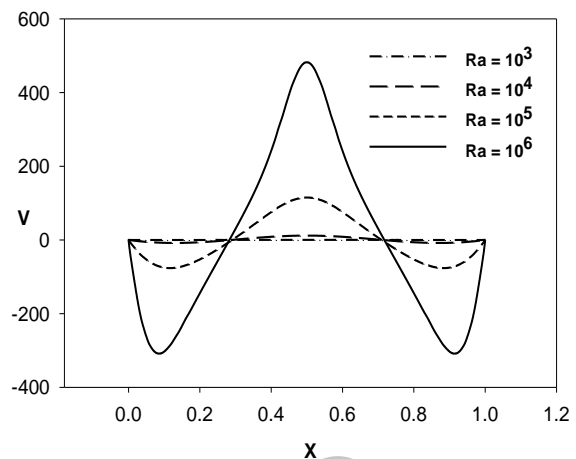
شکل ۴- تغییرات سرعت عمودی به ازای تغییرات ریلی برای نانو سیال \Phi=0.05
