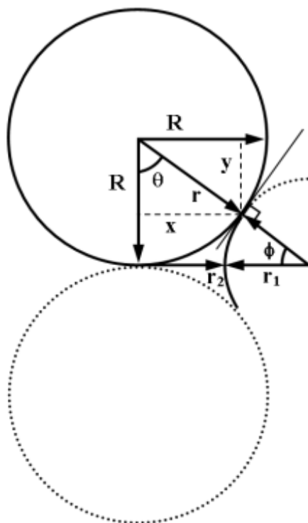
شکل ۱: حجم لنز آب اطراف ذرات کروی از دانه های خاک
