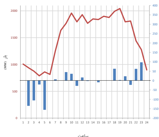
شکل ۷: توان شارژ و دشارژ دستگاه ذخیره‌ساز و بار شبکه در حالت \Delta_1^t = 3 و \Delta_2^t = 1
