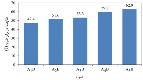
شکل ۵- مقاومت در برابر ضربه پانل‌های کامپوزیتی چوب- سیمان
