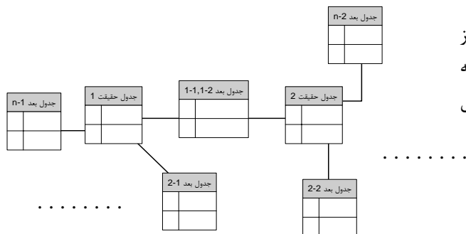
شکل ۳: مدل کهکشانی
