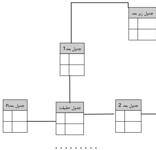
شکل ۶: مدل خوشه‌ستاره‌ای
