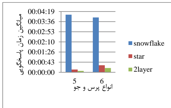
شکل ۱۳: نتایج آزمایشات برای میانگین زمان پاسخگویی در پرس و جوی slice و dice
