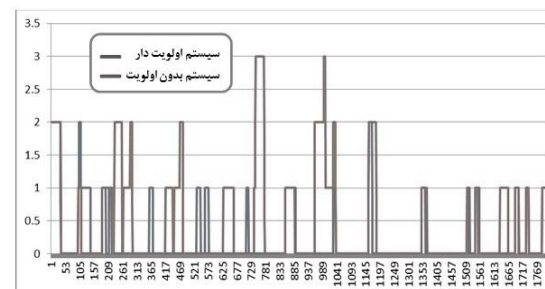
شکل ۵- نمودار مجموع اتوبوس متوقف در چهارراه در هر ثانیه در خیابان شلوغ
