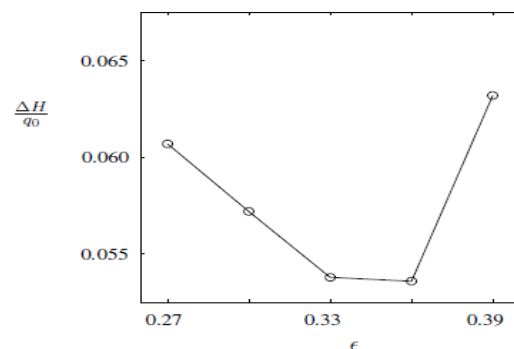
شکل ۳- ضریب افت فشار کل به عنوان تابعی از نسبت باز شونده‌گی (ε) در تحقیقات لیندگرین [۸]
