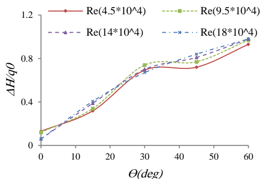
شکل ۱۲- میزان افت فشار کل بر حسب رینولدز در زاویه‌های ورودی مختلف
