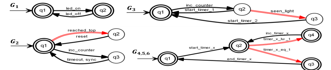
شکل ۱۲: مدل‌های رفتار آزاد ( G_1 تا G_6 ) مربوط به وظیفه همگام‌سازی با استفاده از SCT: x \in \{1, 2, 3\}
