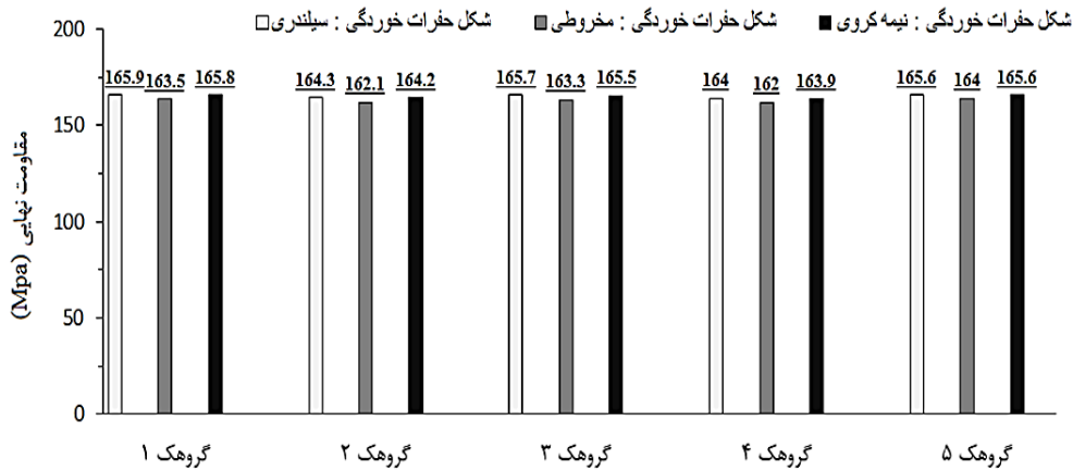
شکل ۶- مقاومت نهایی ورق‌های گروهک‌های پنج‌گانه مربوط به گروه‌های ۱ تا ۳ (ورق‌های فولادی با مقاومت بالا)
