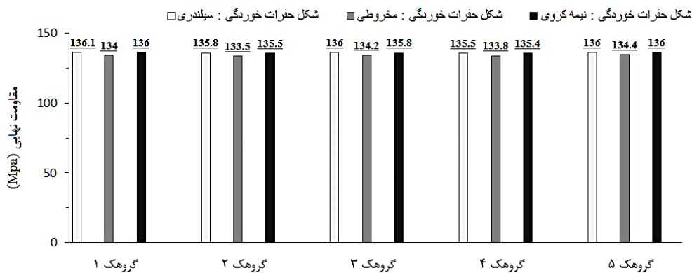
شکل ۷- مقاومت نهایی ورق‌های گروهک‌های پنج‌گانه مربوط به گروه‌های ۴ تا ۶ (ورق‌های فولادی نرمه)
