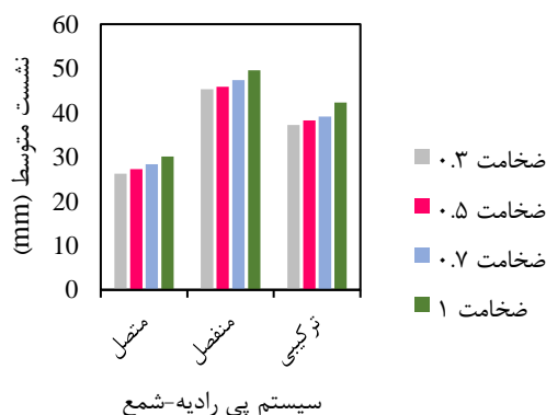
شکل ۱۹: نمودار نشست متوسط رادیه-شمع در ضخامت‌های مختلف رادیه
