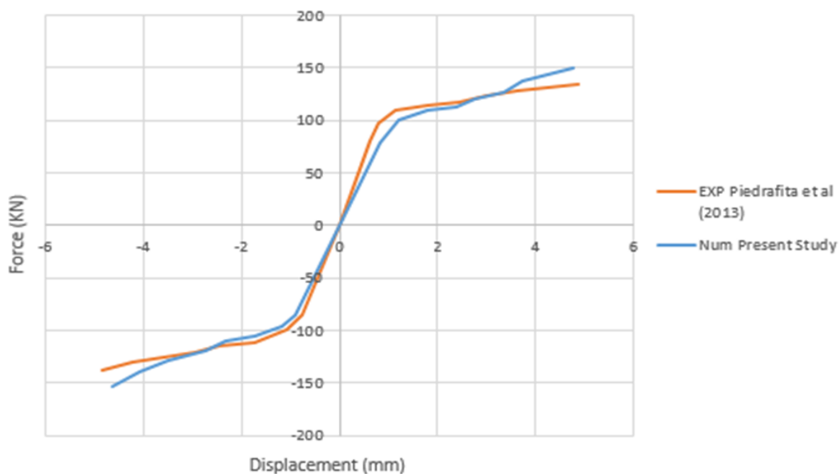
شکل ۱۲- مقایسه پوش نمودار چرخه‌ای آزمایشگاهی در پژوهش پیدرافیتا و همکارانش در سال ۲۰۱۳ [۹] و مدل عددی پژوهش حاضر
