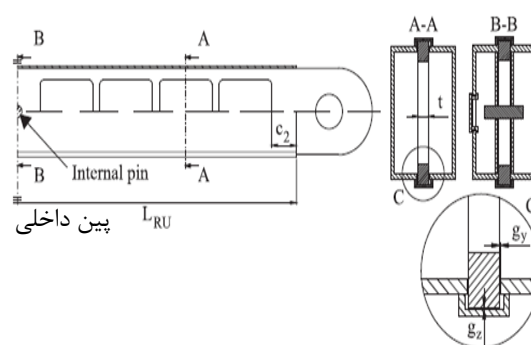
شکل ۲- جزئیات جداگانه یک PCBRB
