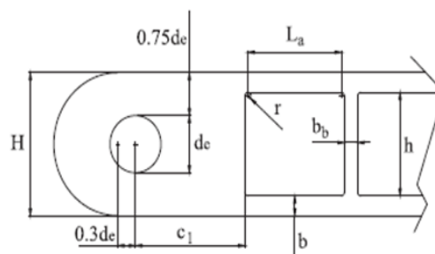
شکل ۳- ابعاد کلیدی هسته PCBRB
