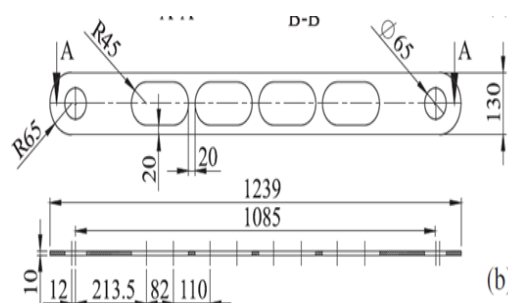
شکل ۴- جزئیات آزمایشگاهی نمونه I
