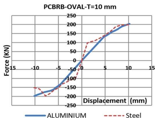
شکل ۱۸- نمودار پوش مدل عددی با هسته آلومینیومی و فولادی
