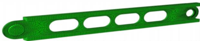
شکل ۹- مدل سازی نمونه پژوهش آزمایشگاهی در پژوهش پیدرافیتا و همکارانش در سال ۲۰۱۳ [۷]
