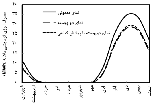
شکل ۷: نمودار مقایسه مصرف انرژی گرمایشی ماهانه
