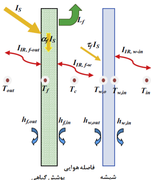
شکل ۵: مکانیزم انتقال حرارت در نمای دو پوسته دارای پوشش گیاهی [۳۴]
