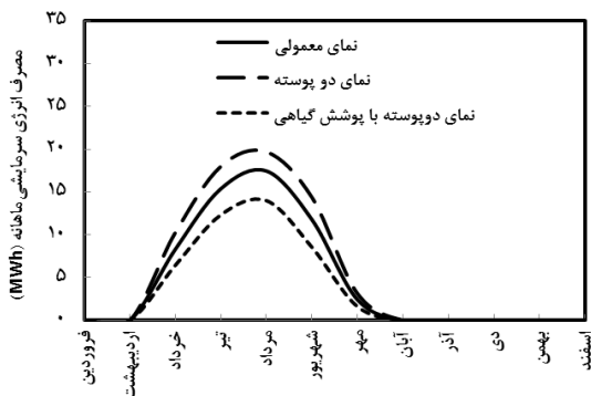
شکل ۸: نمودار مقایسه مصرف انرژی سرمایشی ماهانه
