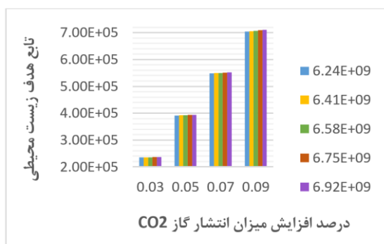
شکل ۵: نمودار میزان تغییرات تابع هدف زیست محیطی به ازای تغییر در میزان انتشار گاز CO 2
