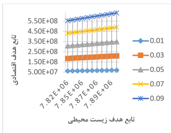
شکل ۴: نمودار پارتو مربوط به افزایش قیمت فروش
