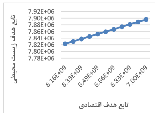
شکل ۳: مرز بهینه پارتو ناشی از حل مسئله
