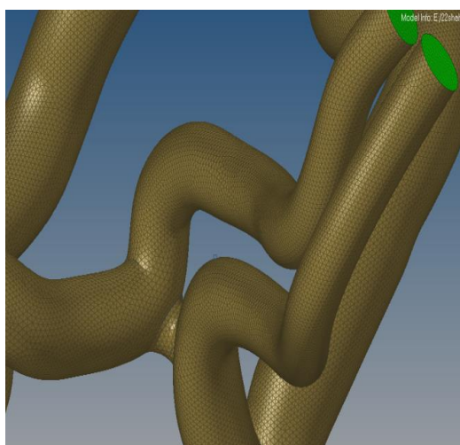
شکل ۴- نمایشی از شبکه‌بندی نهایی سیال
