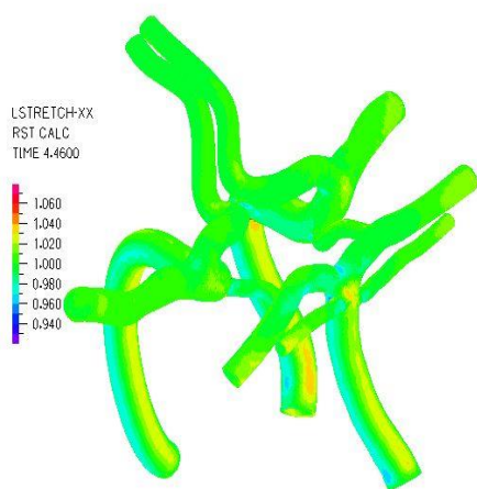
شکل ۱۲- کشیدگی در جهت XX روی دیواره در حالت دیاستول
