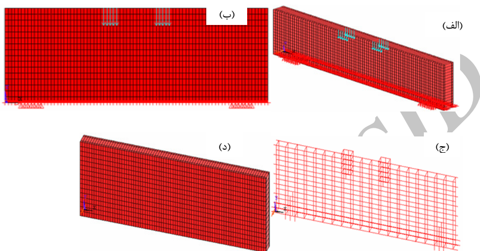
شکل ۱۸- چگونگی مدل‌سازی تیر عمیق بتن مسلح در ANSYS: (الف) شبکه بندی و بارگذاری تیر به صورت سه بعدی؛ (ب) شبکه بندی و بارگذاری تیر به صورت دو بعدی؛ (ج) مدل‌سازی اجزای بتن؛ (د) مدل‌سازی میلگردهای فولادی [۲۹].
