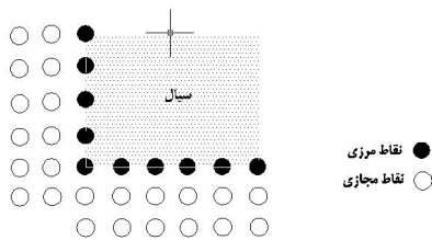
شکل ۳- ذرات مجازی به منظور مدل‌سازی مرز جامد
