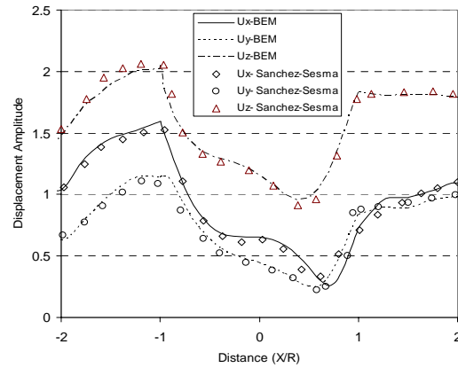
شکل ۵- مقایسه نتایج به دست آمده از تحلیل عددی و نتایج ارائه شده توسط سانچز سسما [۱۳] برای موج ورودی P با زوایای برخورد افقی و قائم ۴۵ و فرکانس بی بعد ۰/۵ برای دره نیم دایره‌ای منشوری
