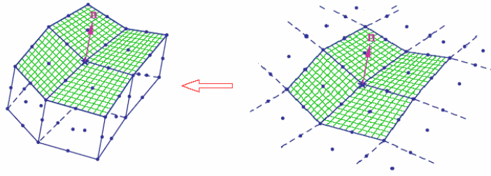
شکل ۳- تبدیل مسئله نامحدود با استفاده از اجزای محصور کننده به مسئله مشابه محدود در حالت سه بعدی
