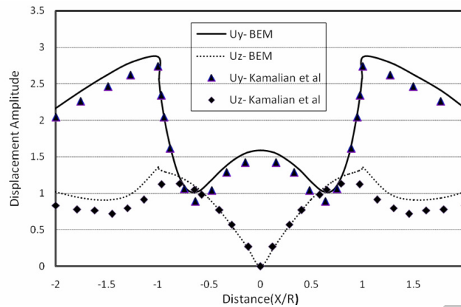
شکل ۷- مقایسه نتایج به دست آمده از تحلیل عددی و نتایج ارائه شده توسط کامالیان و همکاران [۳] برای موج ورودی SV با \theta_h = 90^\circ ، \theta_v = 0^\circ و فرکانس بی بعد نیم برای دره نیم دایره منشوری
