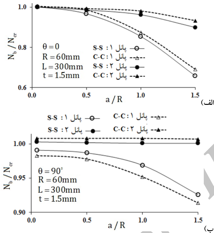
شکل ۷- اثر نوع تکیه‌گاه و زاویه ترک بر بار کمناش فشاری پانل‌ها، الف) با ترک محیطی ب) با ترک محوری
