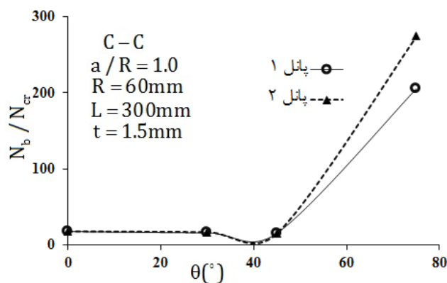
شکل ۱۲- اثر امتداد ترک بر بار کماتش محوری کششی با تکیه گاه گیردار
