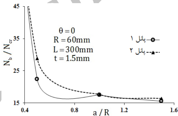
شکل ۱۱- تغییرات بار کماتش کششی بر حسب طول ترک در پانل با تکیه گاه گیردار
