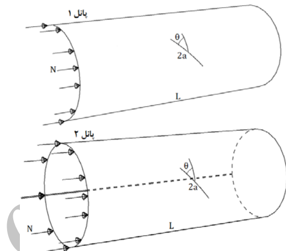
شکل ۲- پانل نیم استوانه (پانل ۱) و استوانه کامل باز (پانل ۲)
