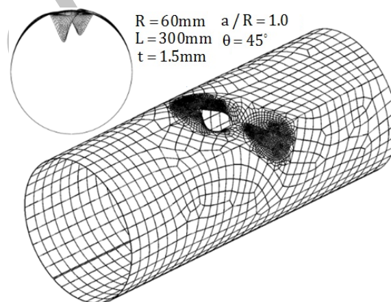
شکل ۴- مود اول کمانش کششی در پانل ۲ با ۳۴۶۶ المان
