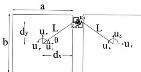
شکل ۴- مختصات قرارگیری فنرهای عمودی و برشی برای دو المان افقی
