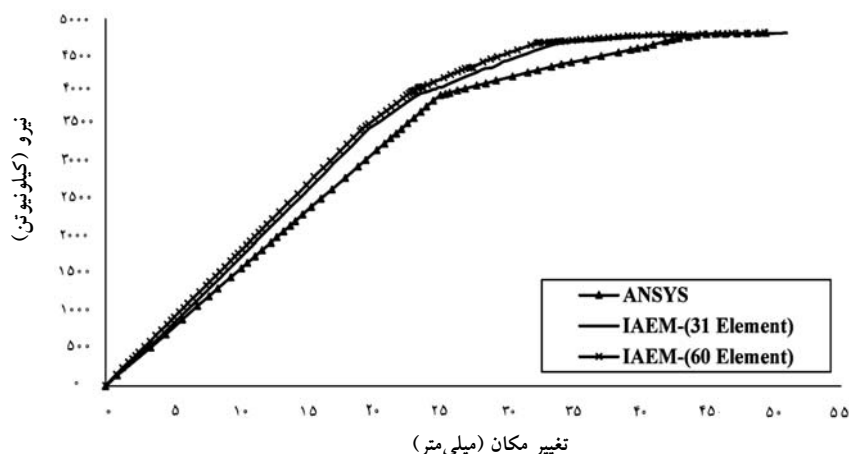
شکل ۱۴- منحنی نیرو- تغییر مکان قاب بتنی در روش‌های تحلیلی IAEM و FEM
