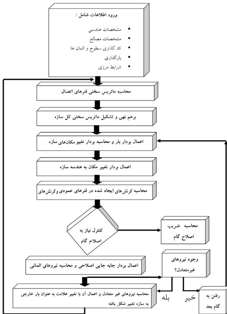
شکل ۸- فلوجارت نرم افزار AEM-SOFT برای تحلیل سازه به روش اجزای مجزای اصلاح شده
