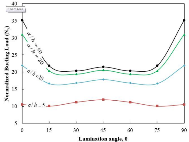
شکل ۶- ضربید بدون بعد کمانش در مقابل زوایای مختلف الیاف یک ورق چندلایه ارتوتروپیک مربعی با شرایط مرزی چهار طرف مفصل با ترکیب لایه [\theta^\circ / -\theta^\circ] برای نسبت بعد به ضخامت a/h مختلف و مدول الاستیسته E_1/E_2 = 40
