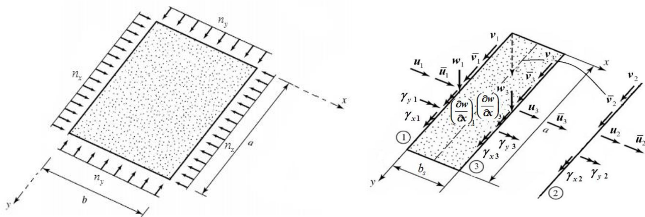
شکل ۱- المان نوار محدود و درجات آزادی در خطوط گروه‌ای یک المان
