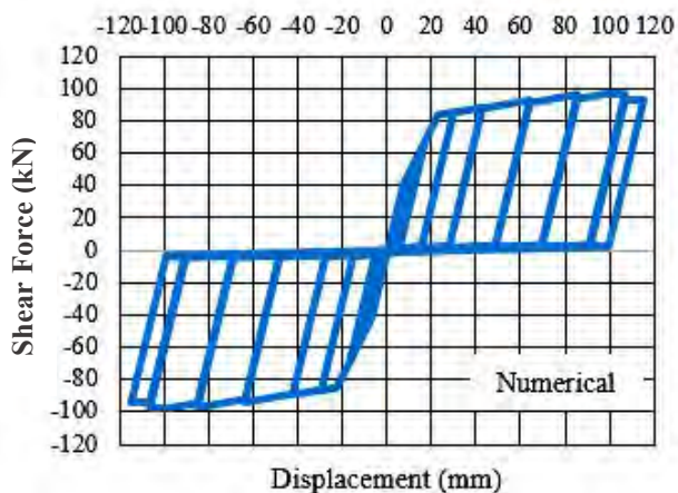
شکل ۱۲- نتایج صحت‌سنجی مدل‌های عددی قاب‌های با تسمه بادبندی تحت بار رفت و برگشتی با نتایج آزمایشگاهی: الف) نمونه 83A-C لوو [۱۵]، ب) نمونه نمونه EA1 حاتمی و همکاران [۱۴]، ج) نمونه 38A-C ولچو [۸]
