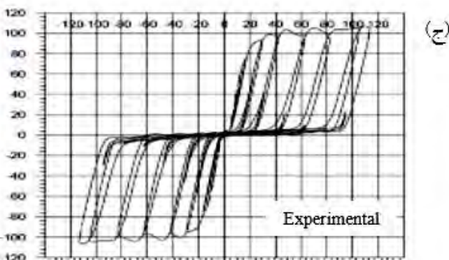
شکل ۱۲- نتایج صحت‌سنجی مدل‌های عددی قاب‌های با تسمه بادبندی تحت بار رفت و برگشتی با نتایج آزمایشگاهی: الف) نمونه 83A-C لوو [۱۵]، ب) نمونه نمونه EA1 حاتمی و همکاران [۱۴]، ج) نمونه 38A-C ولچو [۸]
