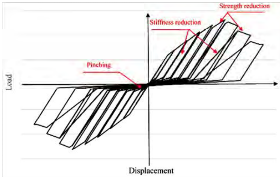
شکل ۱- ویژگی‌های منحنی رفت و برگشتی پل گچی
