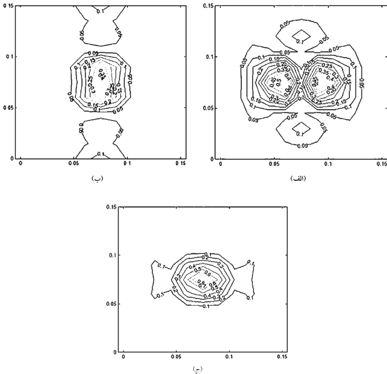
شکل ۱۸- نحوه توزیع شکست با معیار چوی-چانگ در ورق [۹۰/۰/۹۰/۰/۹۰] الف) در سطح بالای لایه اول، ب) سطح پایین لایه چهارم و ج) سطح پایین لایه پنجم
