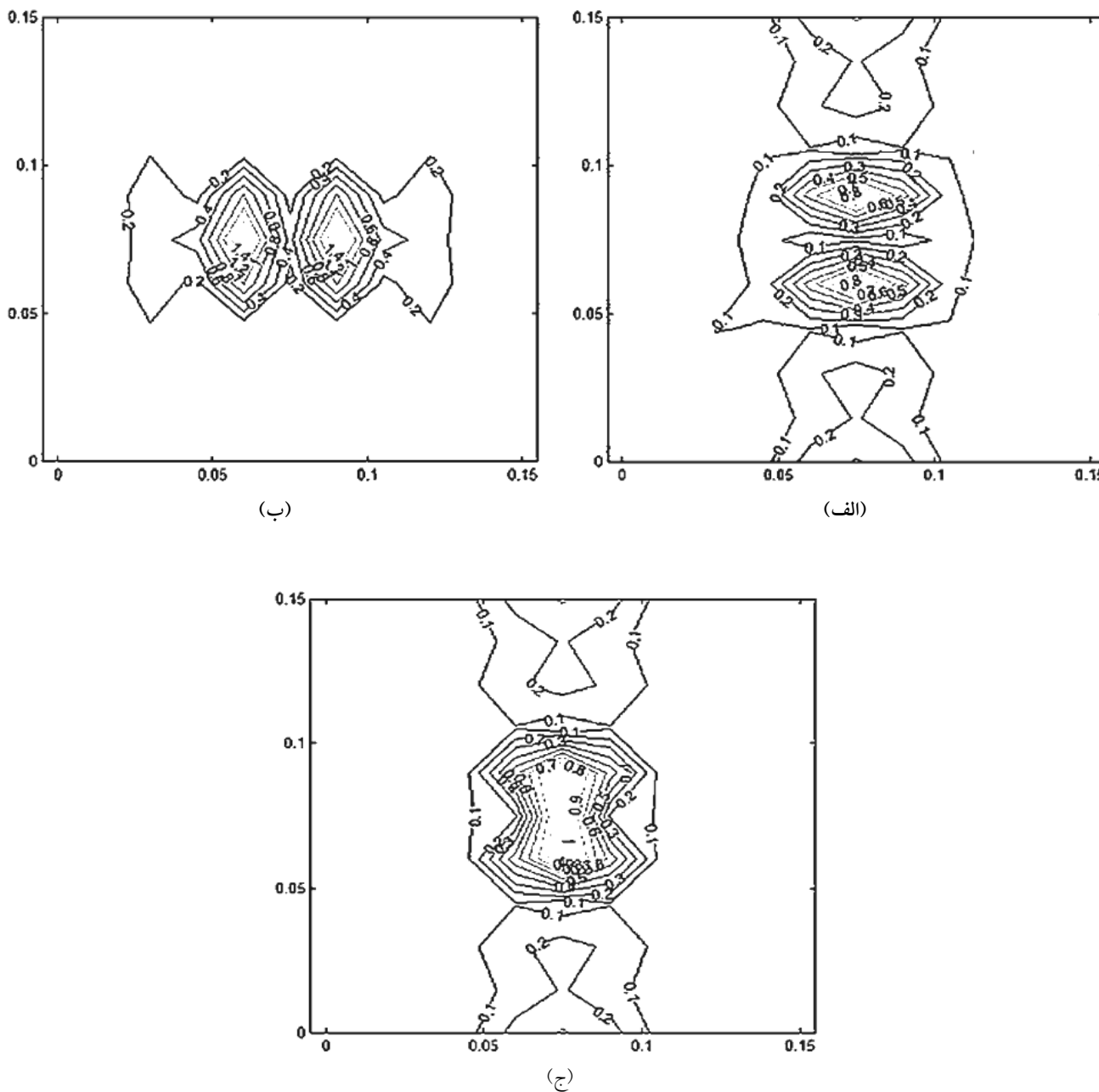
شکل ۱۹- نحوه توزیع شکست لایه لایه شدن با معیار چوی- چانگ بین لایه ها در ورق [۰/۹۰/۹۰/۰/۹۰]: (الف) بین لایه دوم و سوم، (ب) بین لایه سوم و چهارم و (ج) بین لایه چهارم و پنجم
