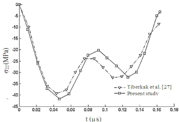
شکل ۵ - تغییرات تنش \sigma_{22} درالمان مرکزی لایه بالایی ورق
