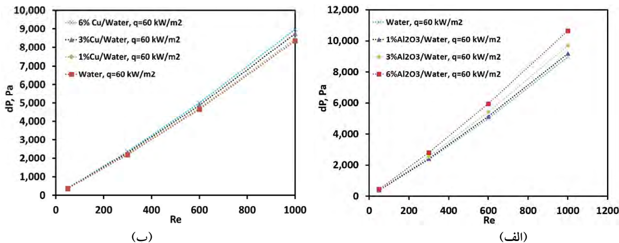
شکل ۸- الف) مقایسه افت فشار نانوسیال ( الف) آلومینا/آب با غلظت‌های ۱، ۳ و ۶ درصد در اعداد رینولدز مختلف و ب) مس/آب با غلظت‌های ۱، ۳ و ۶ درصد در اعداد رینولدز مختلف
