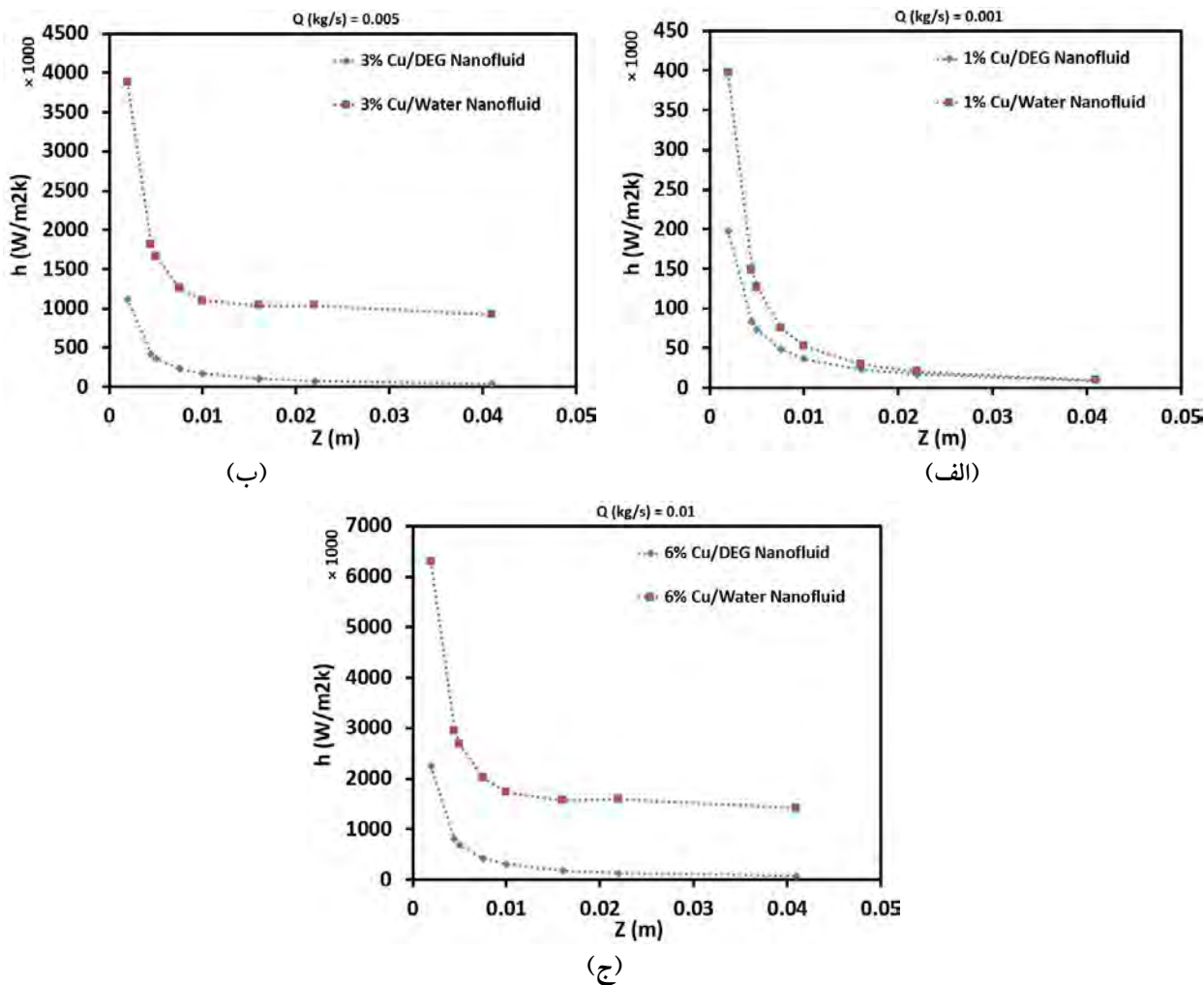
شکل ۱۰- الف) مقایسه ضریب انتقال حرارت جابه‌جایی نانوسیال‌های مس/آب و مس/گلیکول با غلظت: الف) ۱ درصد در دبی جرمی ۰/۰۰۱ کیلوگرم بر ثانیه، ب) ۳ درصد در دبی جرمی ۰/۰۰۵ کیلوگرم بر ثانیه و ج) ۶ درصد در دبی جرمی ۰/۰۱ کیلوگرم بر ثانیه
