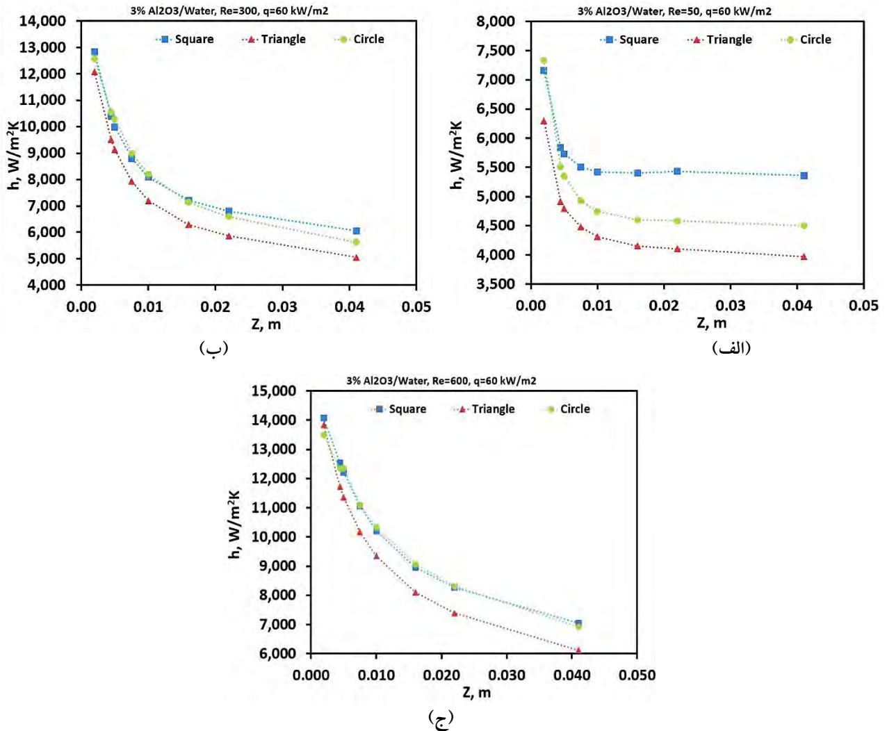
شکل ۵- تأثیر هندسه سطح مقطع میکروکانال بر ضریب انتقال حرارت برای نانوسیال Al_2O_3/water و q=60 \text{ kW/m}^2 : (الف) عدد رینولدز ۵۰، (ب) عدد رینولدز ۳۰۰ و (ج) عدد رینولدز ۶۰۰
