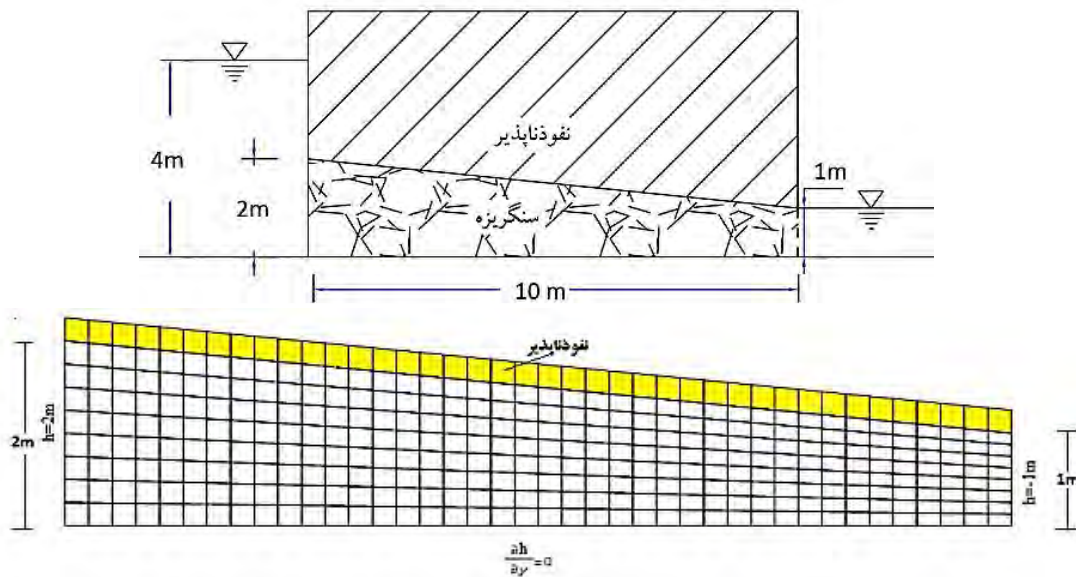
شکل ۱- جریان محدود افقی با سطح مقطع متغیر و شبکه المان محدود به کار رفته به همراه شرایط مرزی حاکم
