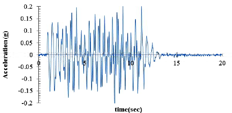
شکل ۴- حرکت ورودی افقی در کف شبکه
