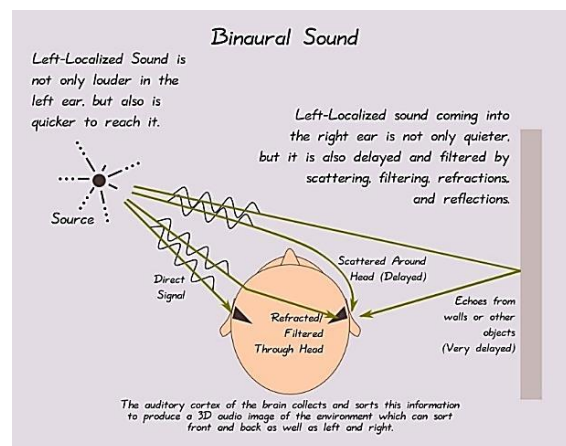
تصویر ۱. شیوهٔ درک فضایی انسان از صدا که سیستم باینورال بر آن مبتنی است مأخذ: Hancock, 2011
