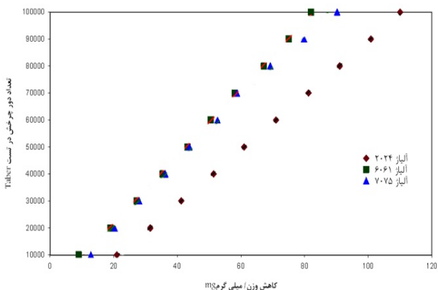
شکل 3- نمودار مقدار کاهش وزن نمونه‌های آزمایش شده بر اساس تعداد دور چرخش آزمایش Taber
