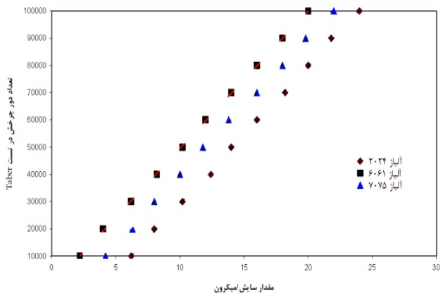
شکل 4- نمودار مقدار سایش بر اساس تعداد دور چرخش آزمایش Taber
