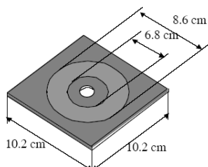
شکل 1- طرح کلی آزمایش سایشی Taber نمونه‌ها
