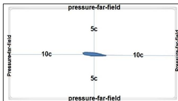
شکل ۱۴- میدان حل عددی
