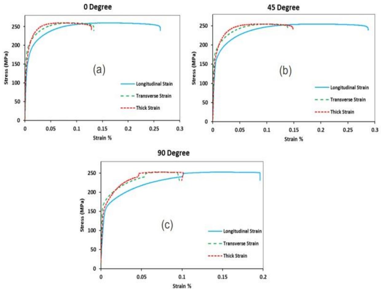
شکل ۱۴ - نمودارهای تنش کرنش مهندسی در کرنش‌های مختلف طولی، عرضی و ضخامتی برای ورق‌های منیزیم در جهات مختلف نورد در (a) زاویه 0 درجه، (b) زاویه 45 درجه، (c) زاویه 90 درجه
