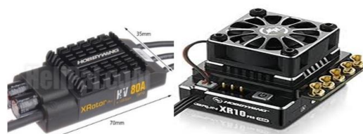
شکل ۱۳- تصویر دو نمونه مبدل و یا کنترل کننده سرعت در موتورهای بدون جاروبک
