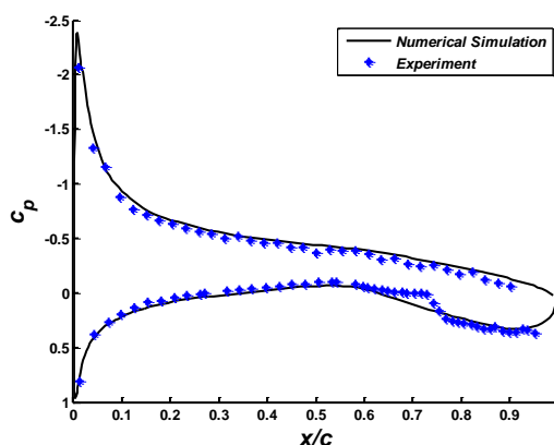
شکل ۸- مقایسه نتایج عددی با تجربی در زاویه حمله ۴ درجه
