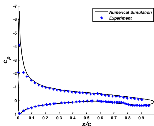
شکل ۹- مقایسه نتایج عددی با تجربی در زاویه حمله ۸ درجه
