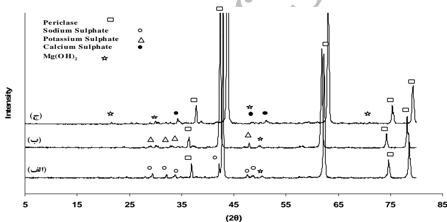
شکل (۴): مقایسه الگوی پراش اشعه ایکس نمونه‌های سولفات با خاصیت بازی در دمای ۱۱۰°C (الف) نمونه SoS، (ب) نمونه PoS و (ج) نمونه CaS.
