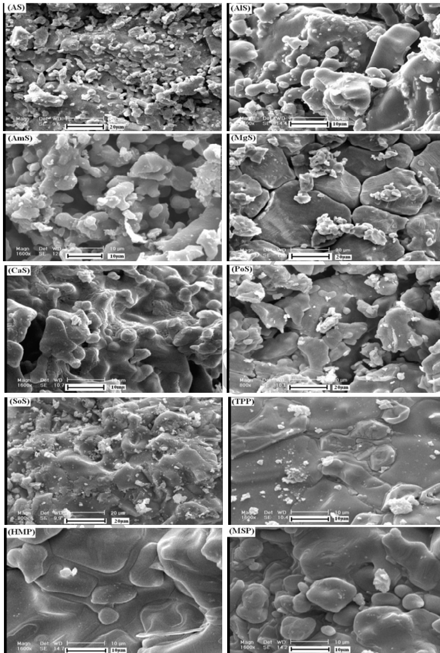
شکل (۵): تصاویر SEM نمونه‌های حرارت دیده در دمای 1400^{\circ}\text{C} به مدت ۳ ساعت.
