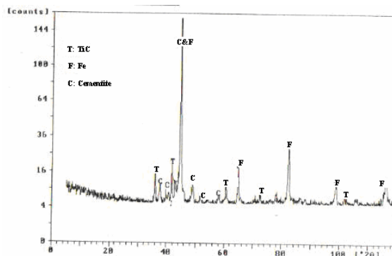
شکل (۳): الگوی پراش اشعه ایکس نمونه AC.
