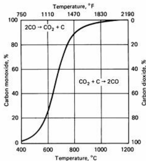
شکل (۱): رابطه نسبت تعادلی CO و CO 2 با دما برای واکنش
