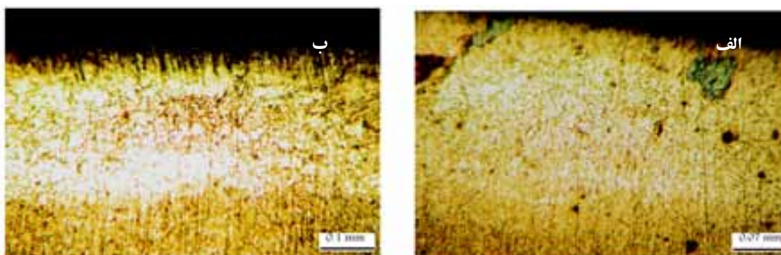
شکل (۵): تشکیل منطقه دکربورگی در لبه نمونه‌های کربوره شده در محفظه دارای فاصله هوایی در زمانهای (الف) ۸ ساعت و (ب) ۱۲ ساعت.
