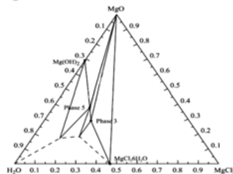
شکل (۱): دیاگرام فازی سیستم سه تایی MgO-MgCl_2-H_2O در دمای اتاق [۷]
