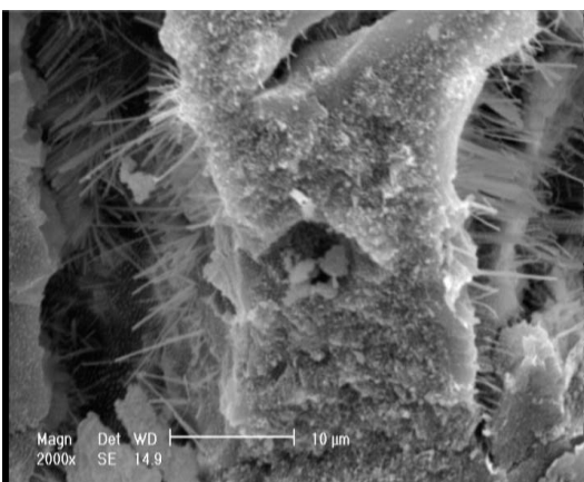
شکل (۳): جوانه زنی فازهای کریستالی سوزنی شکل از درون تخلخل برای
