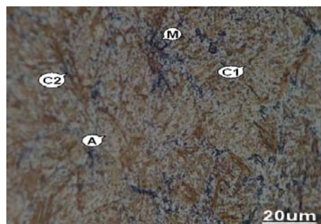
شکل (۶): ساختار فلز رسوب WD در لایه سوم حاوی مارتنزیت (M)، آستنیت (A) و کاربیدهای از نوع MC_1 و M_3C_2
