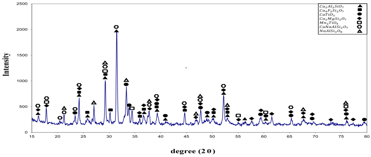
شکل (۷): الگوی XRD نمونه T (ب)
