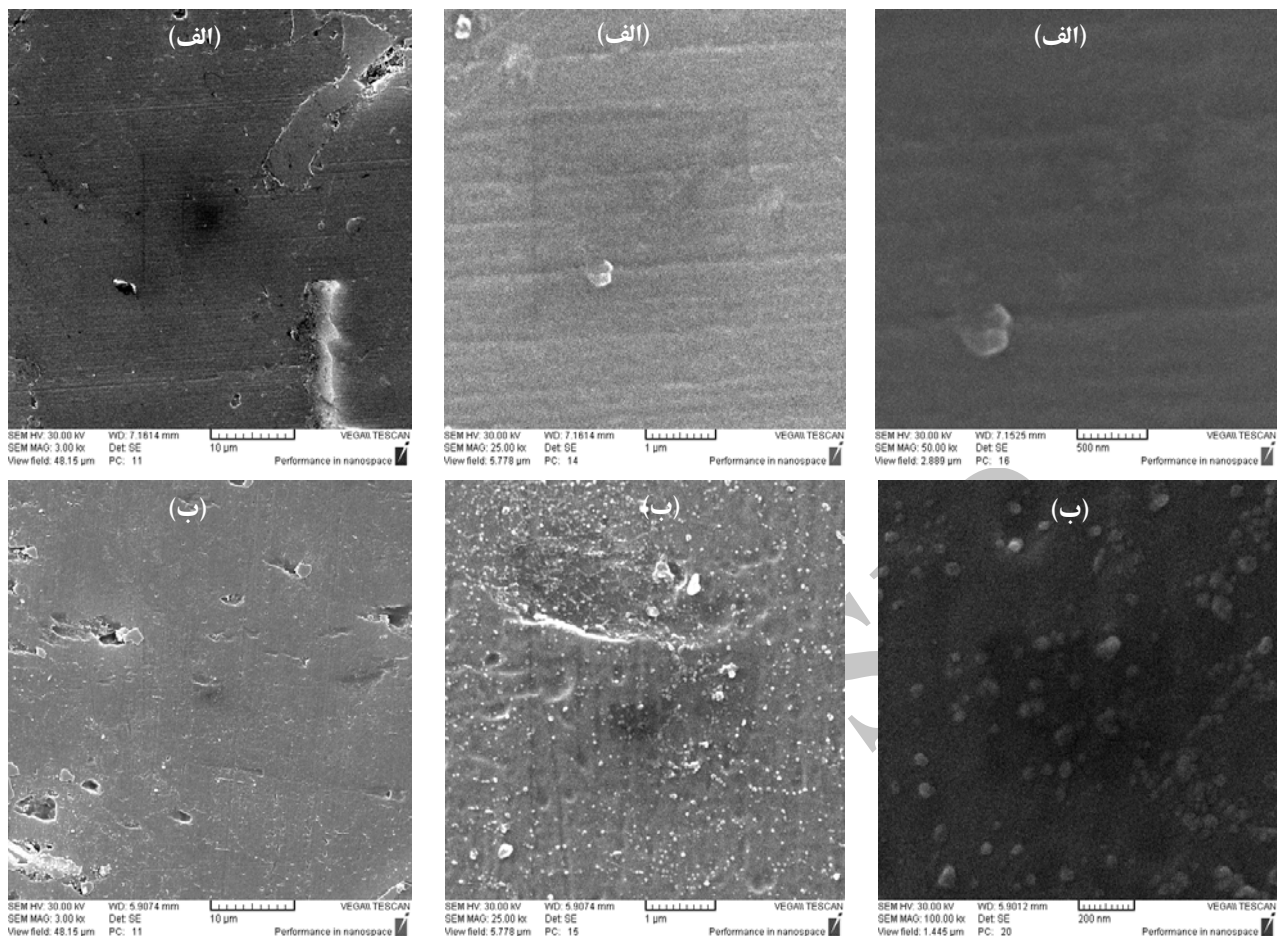
شکل (۲): تصاویر SEM از ریزساختار نمونه‌های مرجع تهیه شده از طریق افزودن: (الف) نانوذرات خام و (ب) پودر آمیژان به مذاب آلیاژ.
