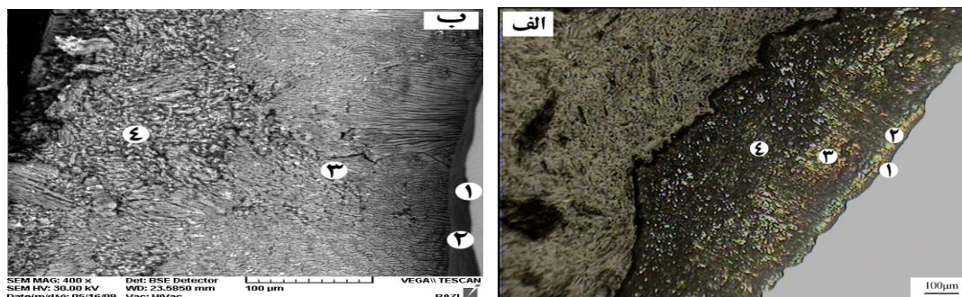
شکل (۴): ریزساختار پوشش ایجاد شده بر روی فولاد 316 غوطه ور شده درون روی 2 برای مدت زمان غوطه وری 120 ساعت در دمای 458°C: الف) میکروسکوپ نوری، نقطه ۱: فصل مشترک فولاد و پوشش، نقطه ۲: گاما، نقطه ۳: دلتا، نقطه ۴: زتا و ب) میکروسکوپ الکترونی
