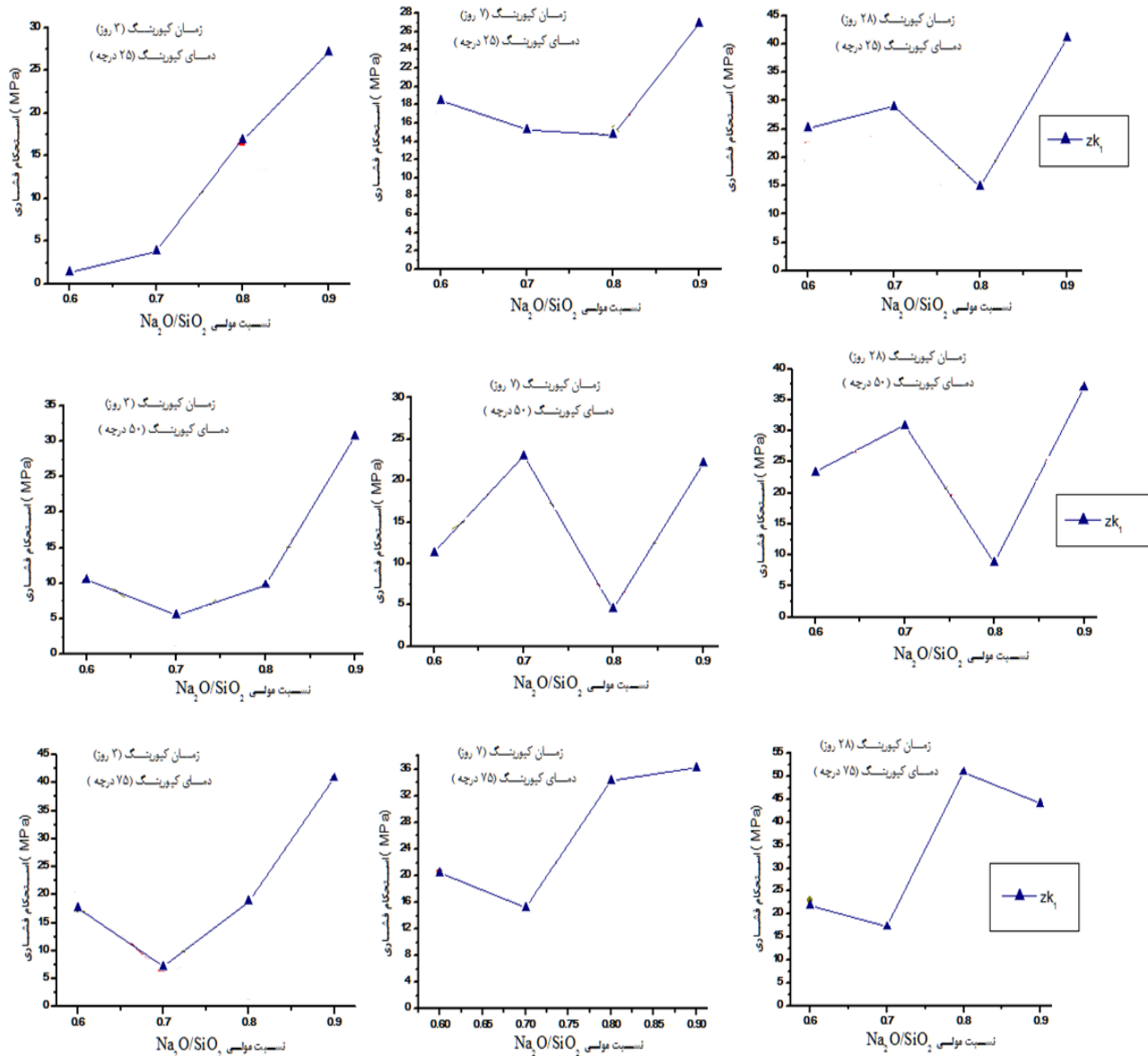
شکل (۴): استحکام فشاری نمونه‌های ژئوپلیمری با نسبت مولی مختلف Na 2 O/SiO 2 فعال کننده در دماهای کیورینگ ۲۵°C و ۵۰°C و ۷۵°C و زمان کیورینگ ۳، ۷، ۲۸ روز و ۲۸ روز
