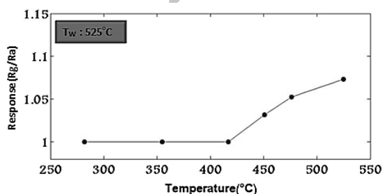
شکل (۴): منحنی تغییرات پاسخ به ۲۰۰۰ ppm گاز اتانول بر حسب دما برای نمونه ۱/۵ Ni-YSZ (دمای کار حسگر: Tw)
