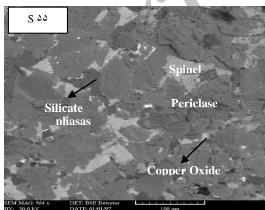
شکل (۳): تصاویر BSE از سطح نمونه‌ها بعد از آزمون بوتنه
