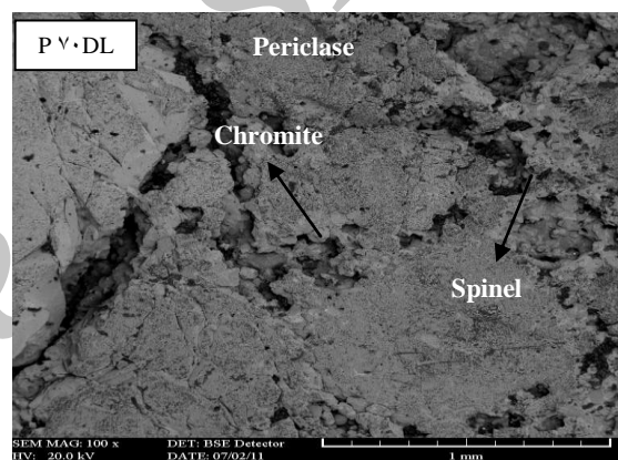
شکل (۲): تصاویر SEM از سطح نمونه‌ها قبل از آزمون بوتنه
